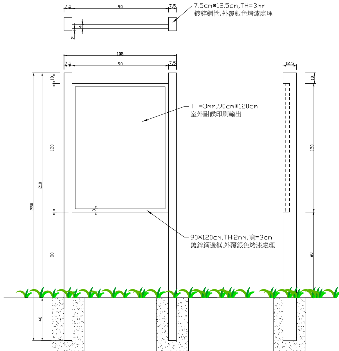
正立面圖
