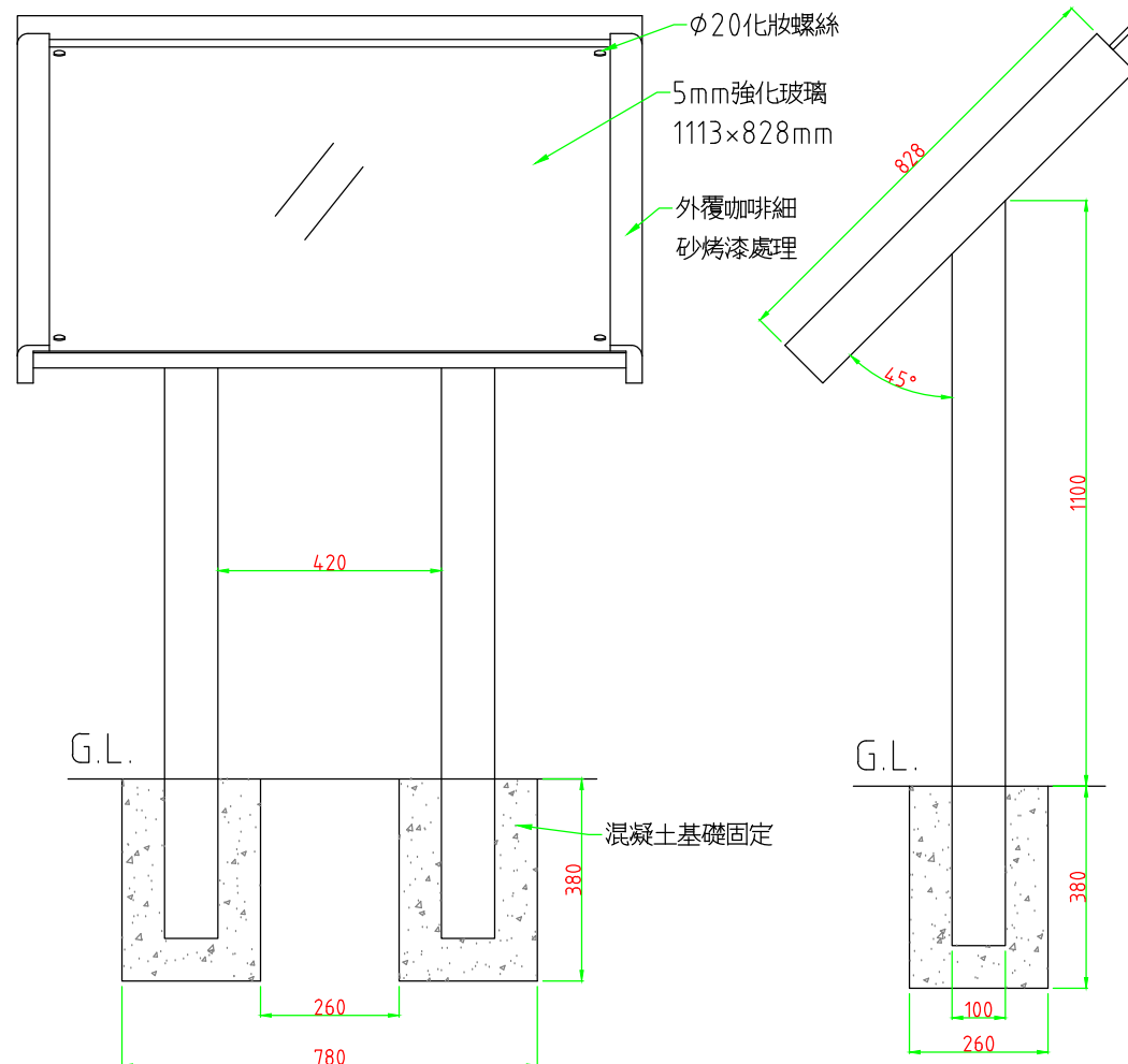
正視圖
