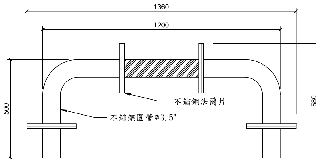
立面圖
