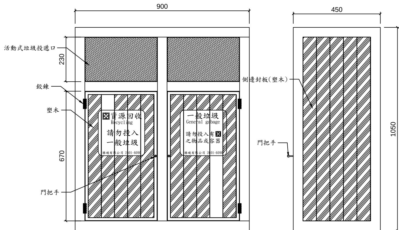
立面圖
