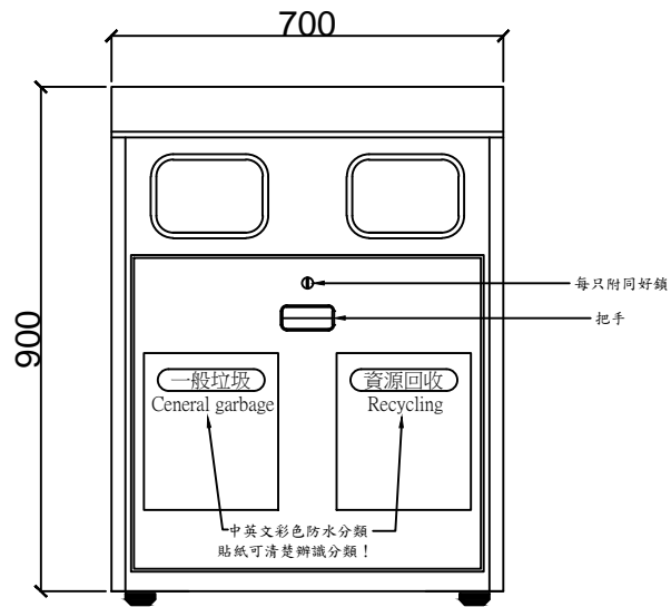
立面圖
