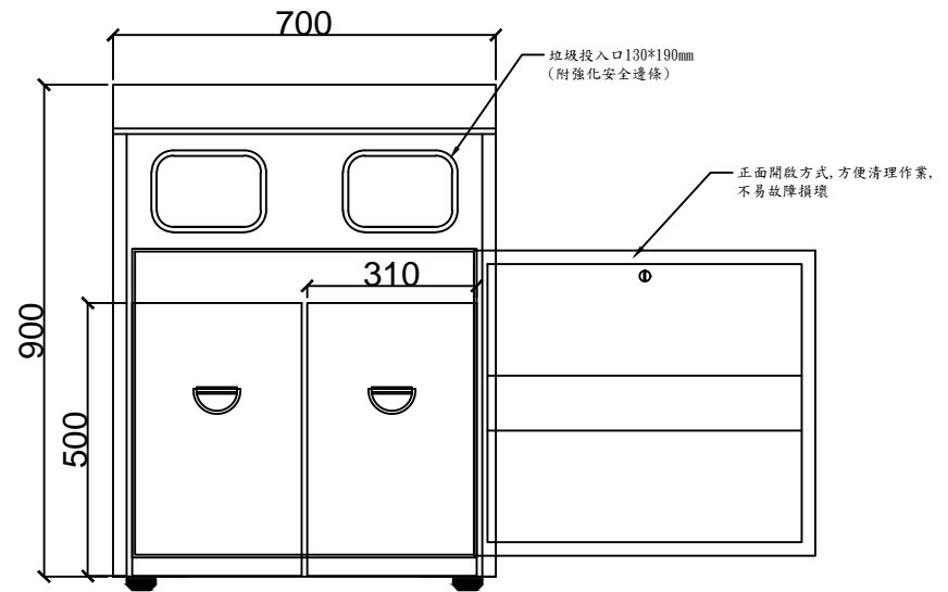
斷立面圖
