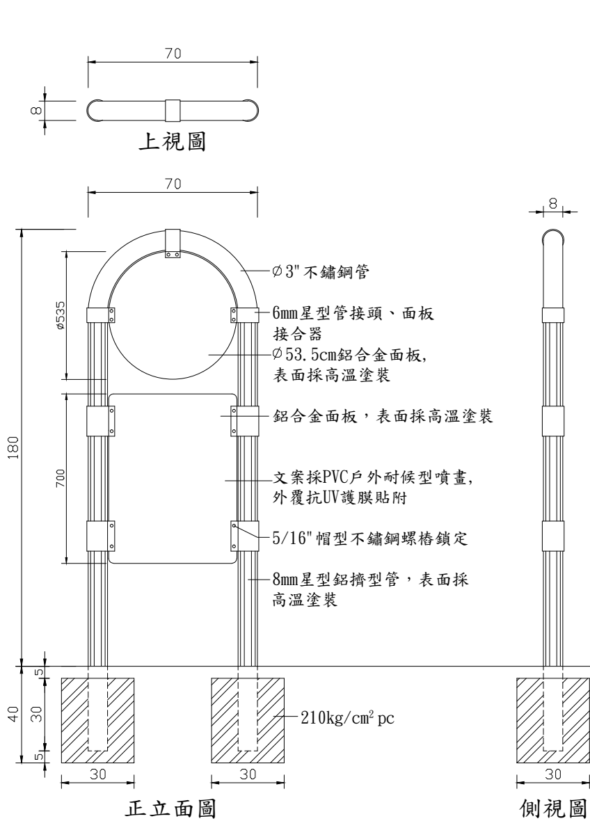
兒童遊戲場告示牌 S=1:20 U=CM
