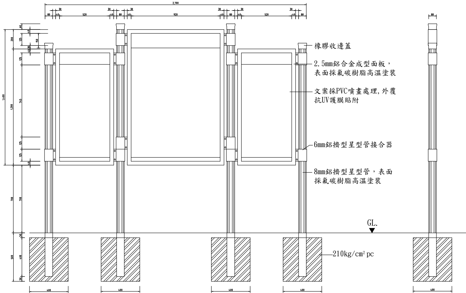
正立面圖
