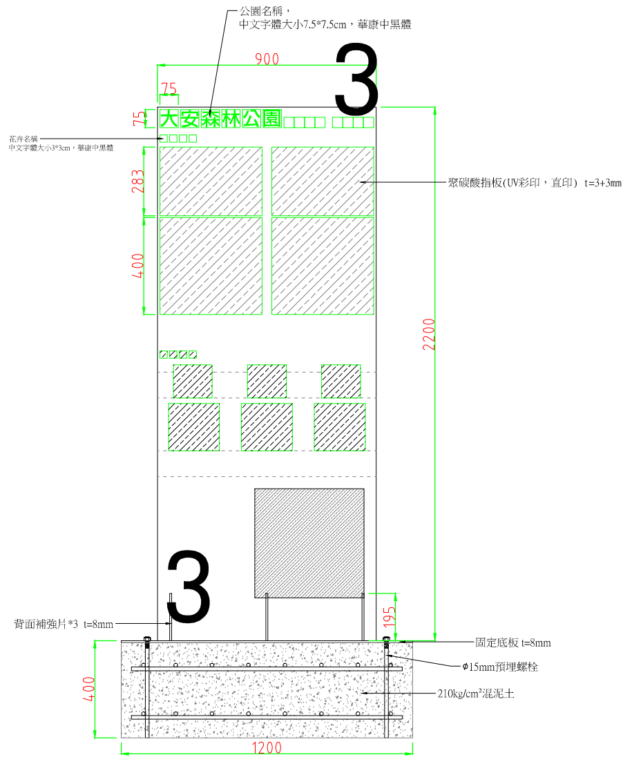
正立面圖
