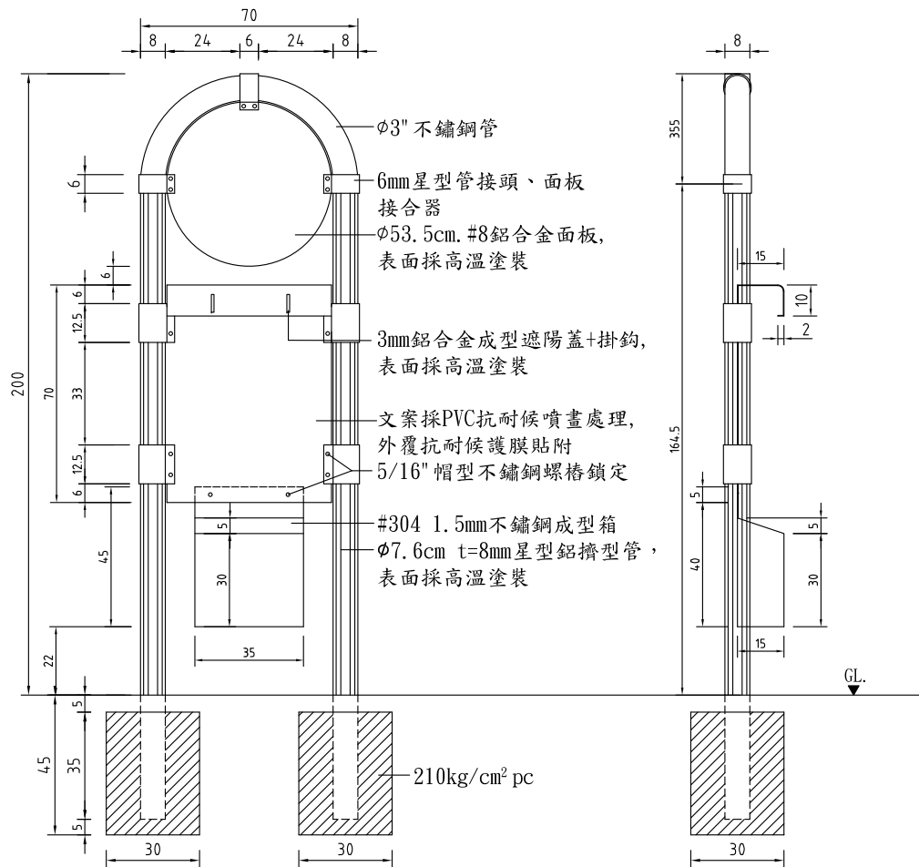
正立面圖
