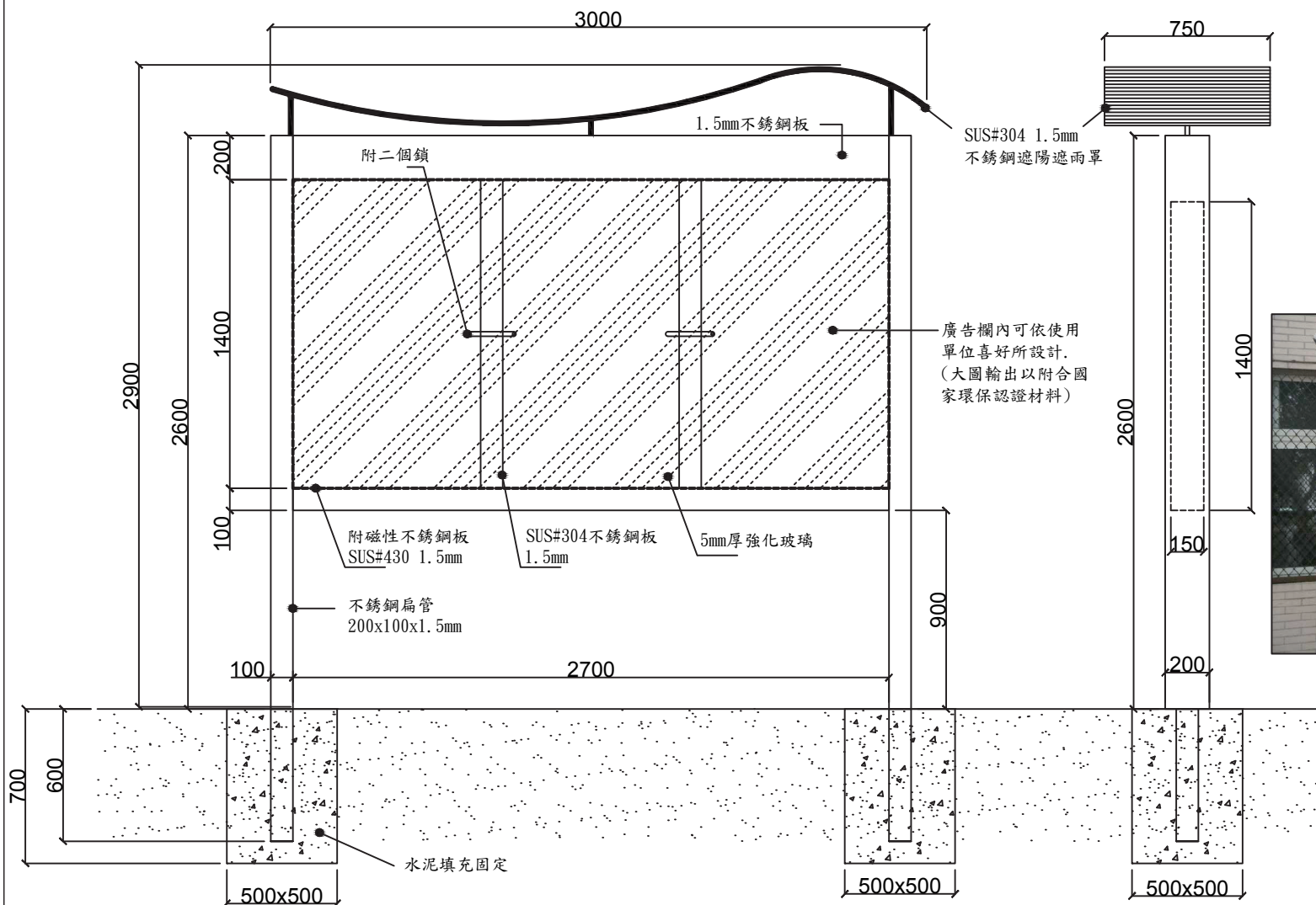
立面圖
