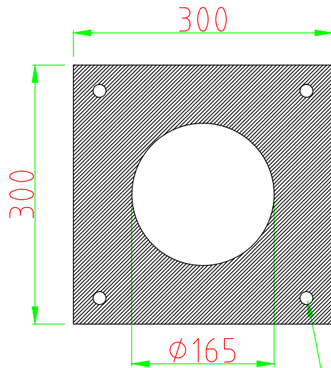
平面圖
