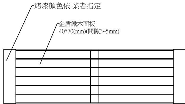
木座椅平面圖
