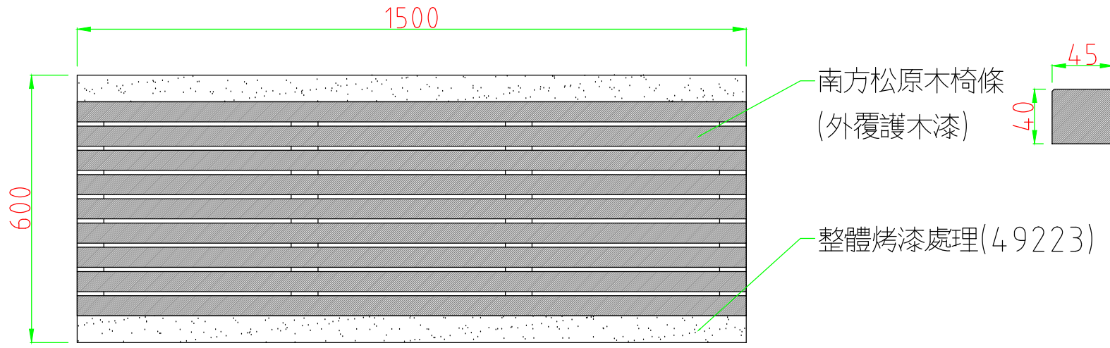
平面圖
