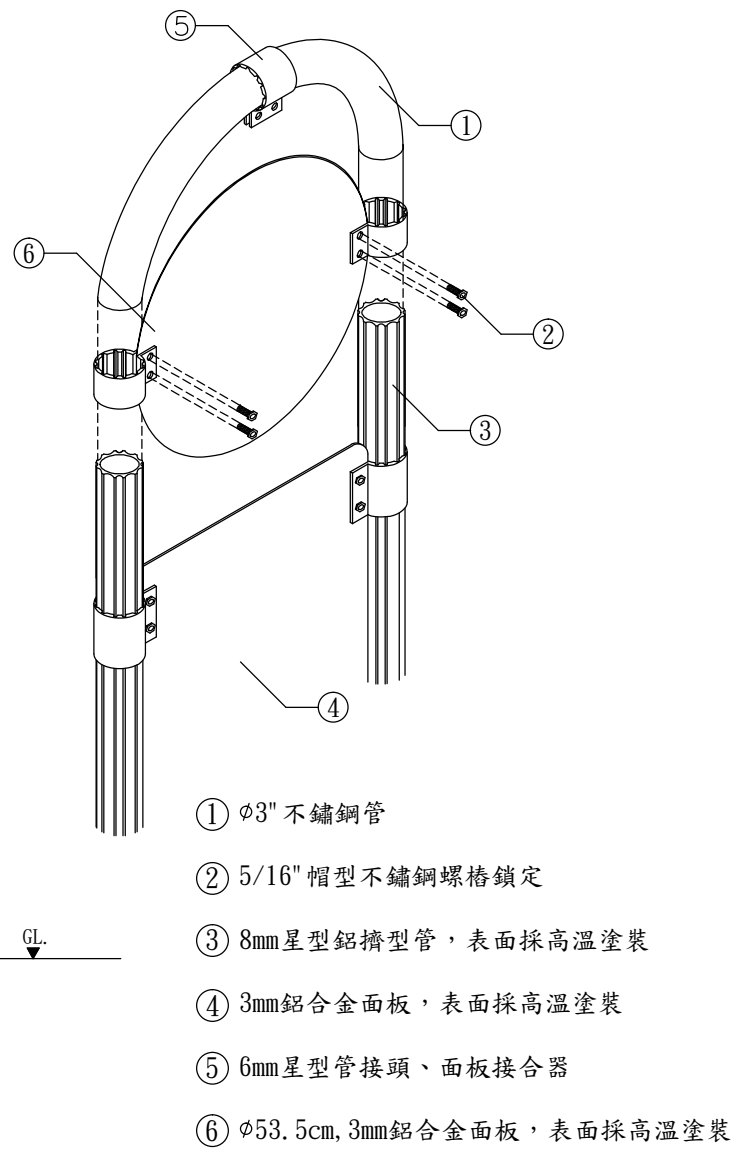
面板接合詳圖
