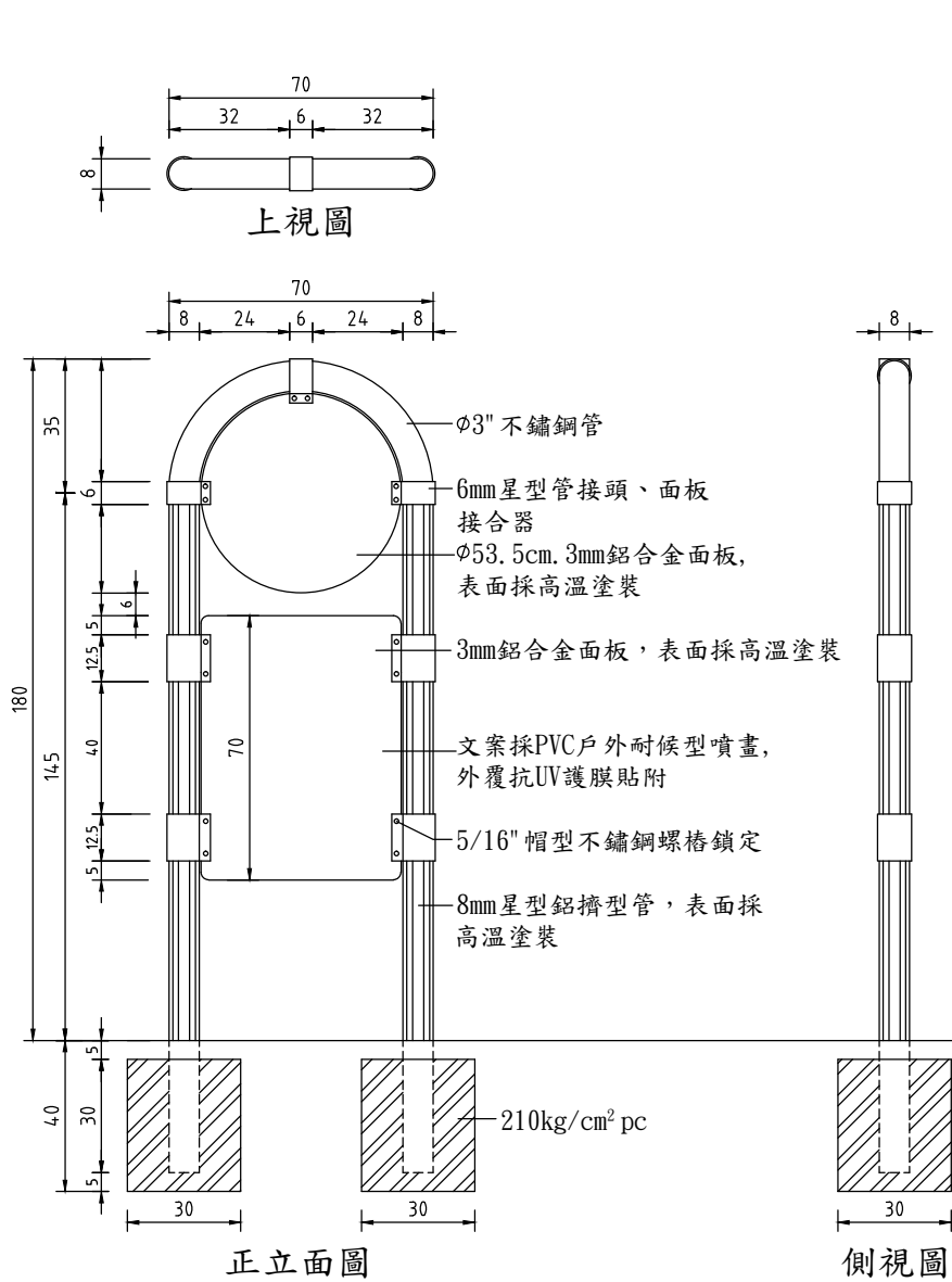
兒童遊戲場標示牌 S=1:20 U=CM
