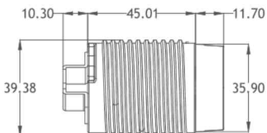
Base Type :Conduction Body(45mm)+Fixer(BX)
