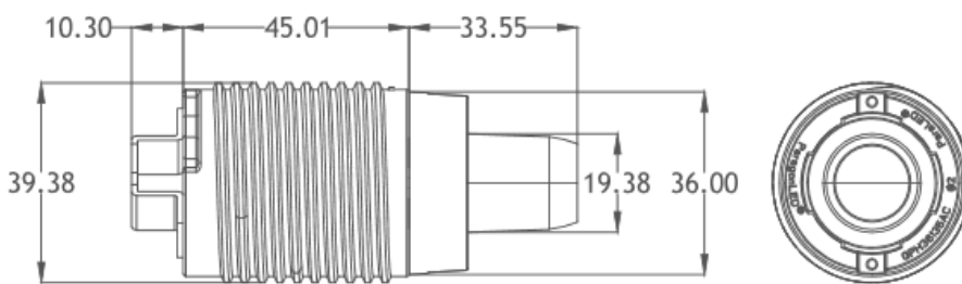
Base Type :Conduction Body(45mm)+Light guide column+Fixer(BB)
