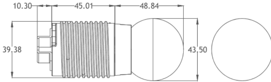
Base Type :Conduction Body(45mm)+Bulb+Fixer(BA)
