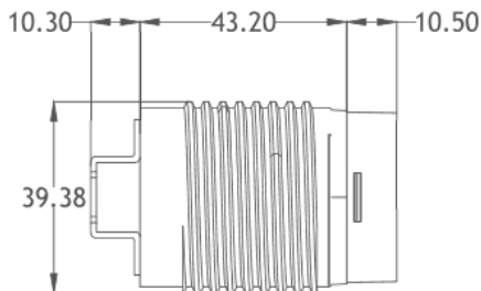
Base Type Conduction Body(45mm)+24° Lens+Fixer(BC) Conduction Body(45mm)+38° Lens+Fixer(BD)
