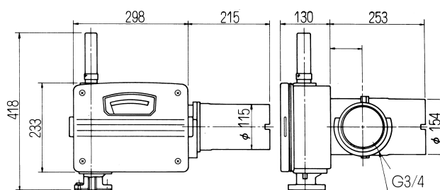
Fig. 10 : FS-115E, 3 and 6 point
